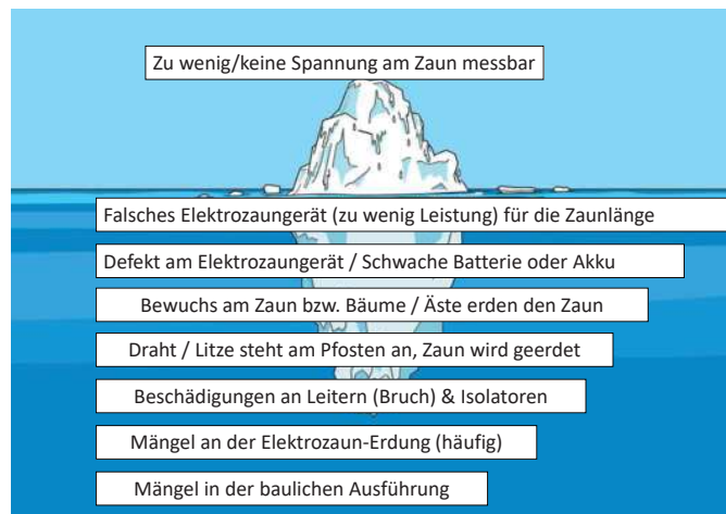
Abb. 10: Schematische Darstellung der auf einander aufbauenden Fehlerursachen.
