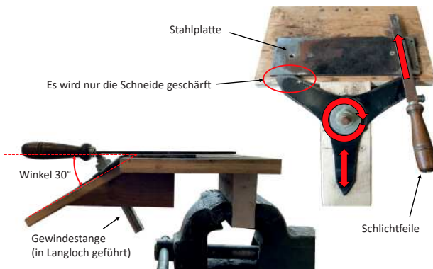
Bild 5: Schärhilfe für Dickichtmesser in Seiten- und Draufsicht (Eigenkonstruktion).
