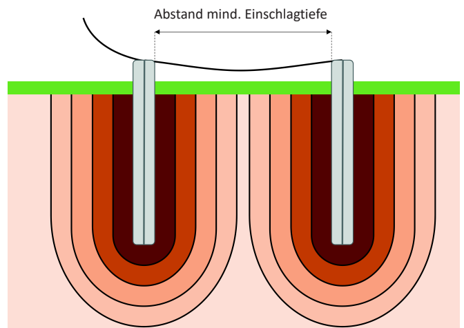
Abb. 18: Schematische Darstellung des Wirkungsbereichs eines Erdungspfahls.
